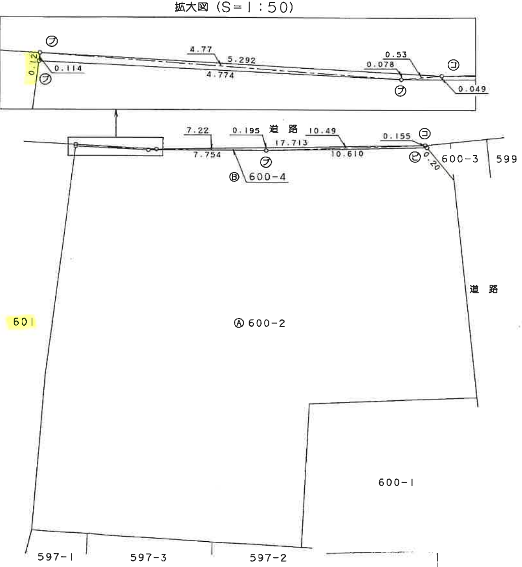
拡大図 (S=1:50)
